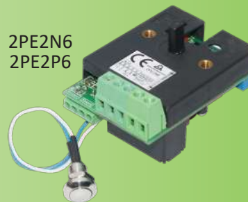
Limitador y termostato electrónico con reinicio manual, rangos de temperatura de hasta 200 °C. Sensor NTC o Pt100.
