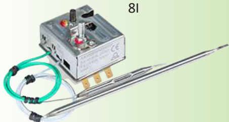
Termostato de reinicio manual de límite alto monopolar, a prueba de fallos, de configuración fija, y rango de temperatura de hasta 320 °C
